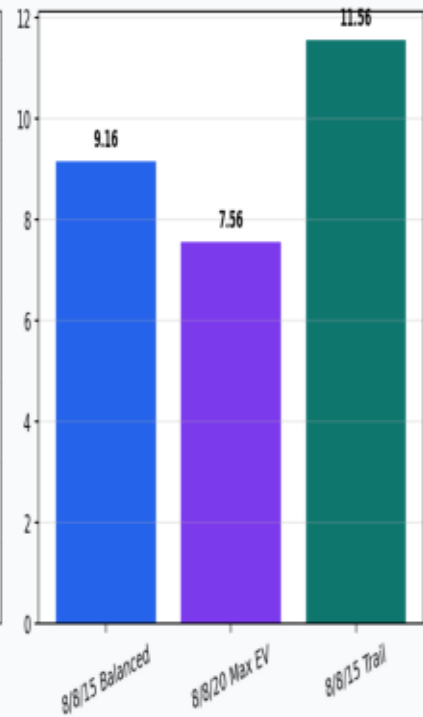
Calmar
